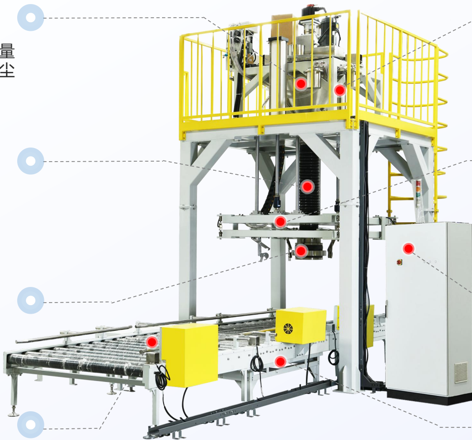
吊钩秤式吨包装机 HEFDZ-1000
