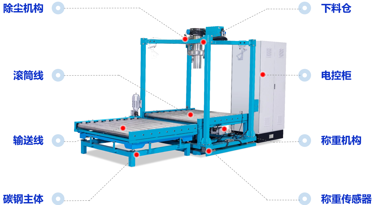
下称重式简易吨包装机 HEFXQ-1000
