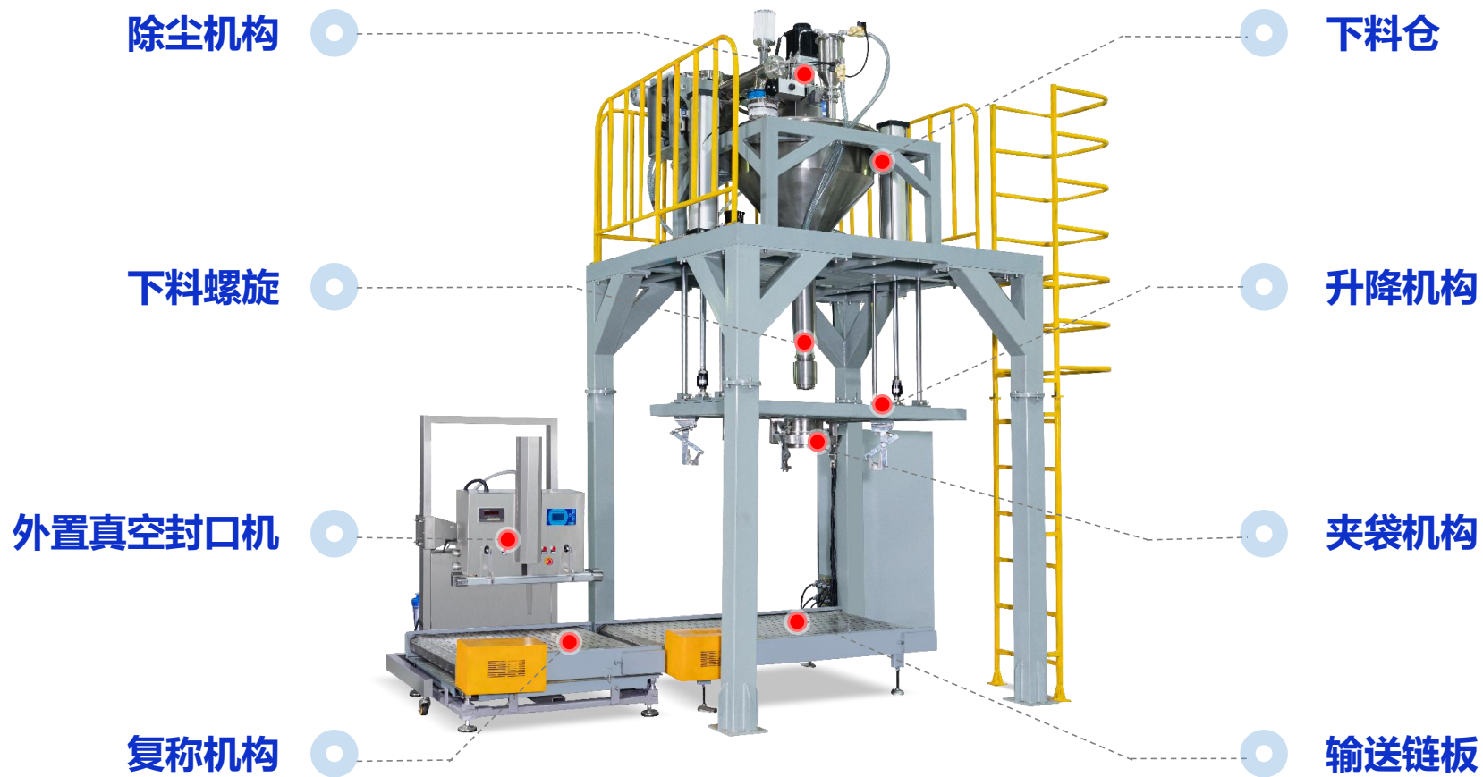
超细粉上称重式吨包机 HEFSZ-1000
