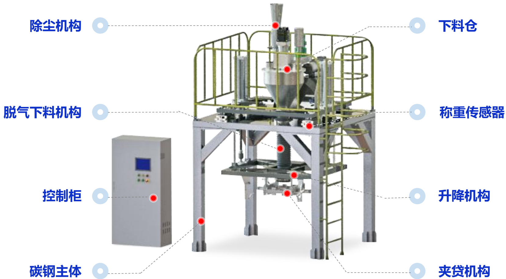
超细粉下称重式吨包机 HEFXZ-1000
