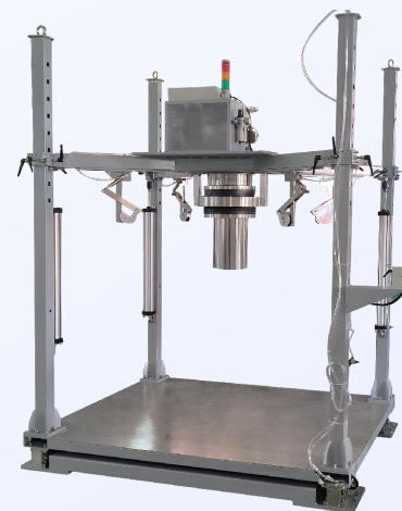
简易吨包机
