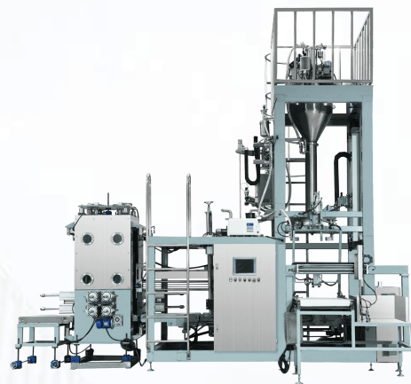
粉料全自动包装机 (1-50kg) HEZ-50
