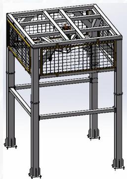
吨包叠包机
