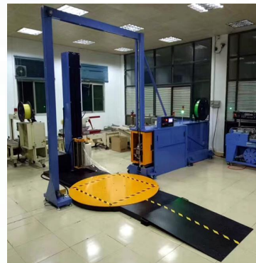
超细粉专用缠绕膜机
