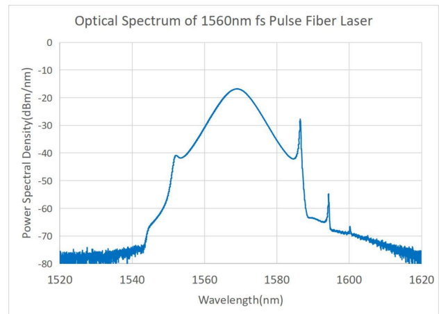
光谱
