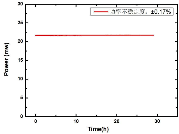
功率稳定性
