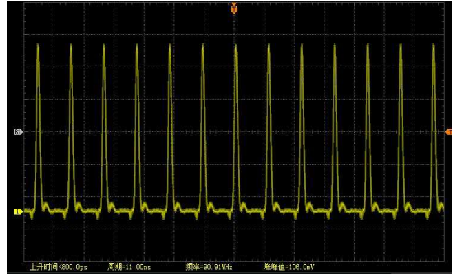
脉冲序列
