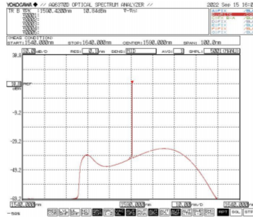
L 波段放大输出光谱(1590nm, 10W 功率)
