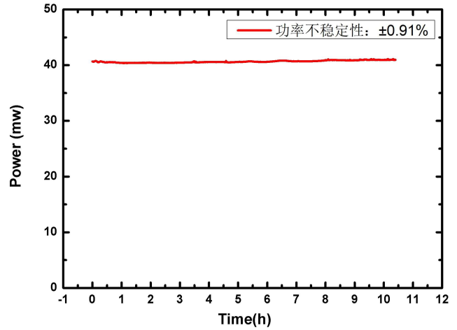
功率稳定性
