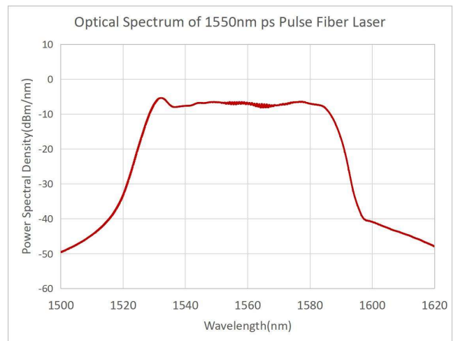
光谱 (宽谱)
