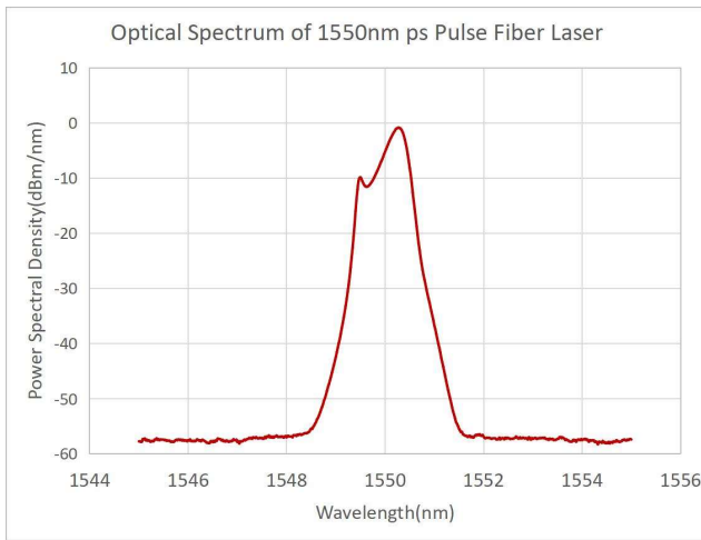
光谱 (窄谱)
