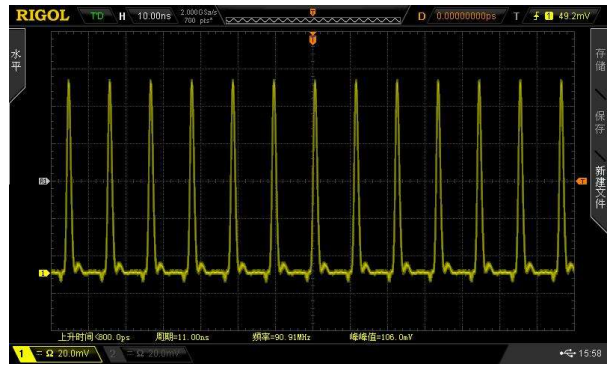
脉冲序列
