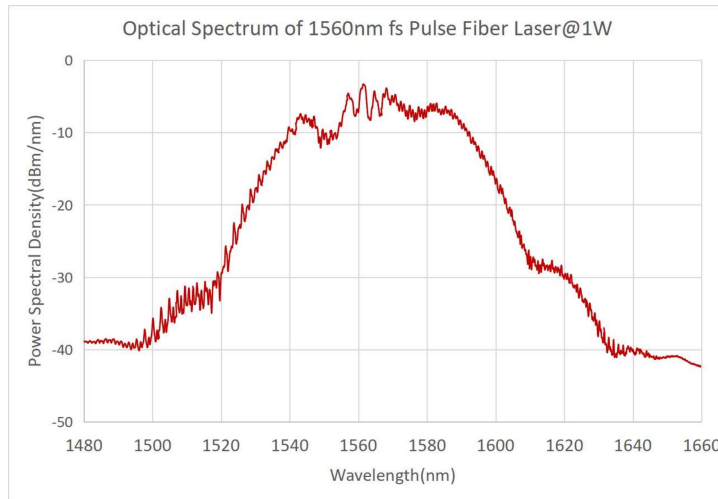
光谱
