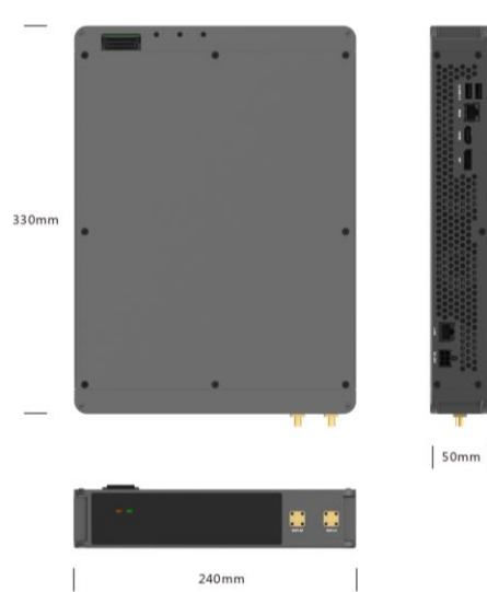
操控模块 SAK1000/WSNs-P
