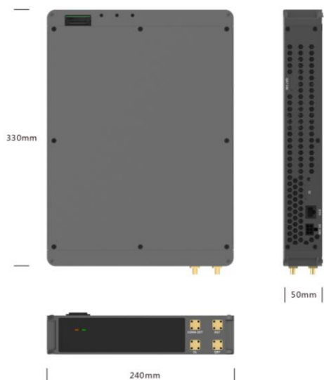
CDMA制式模块 SAK1000/WSN-C
