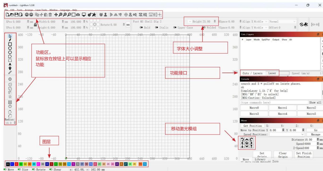
图 30 Lightburn 界面
