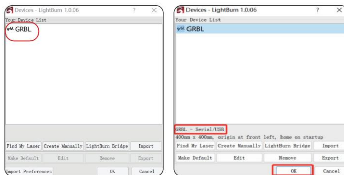
图 27 选择 GRBL
