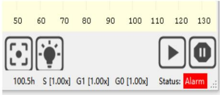
图 9 状态 :报警
