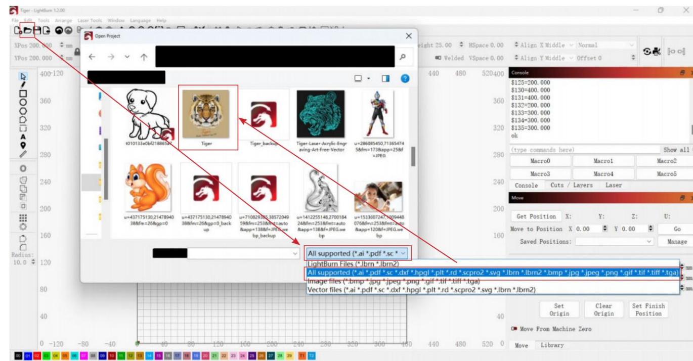
图 31 导入图像
