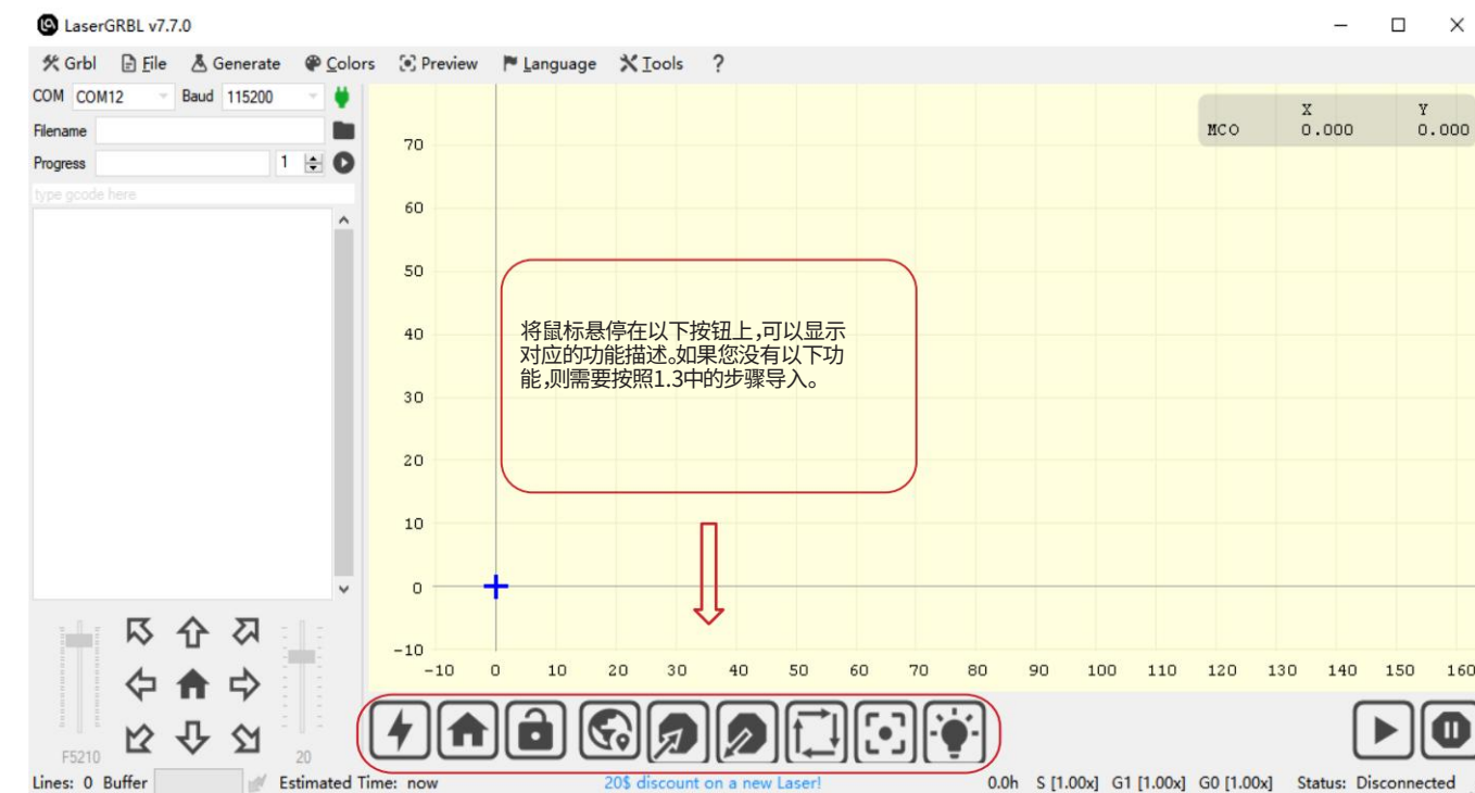
图2 LaserGRBL 界面
