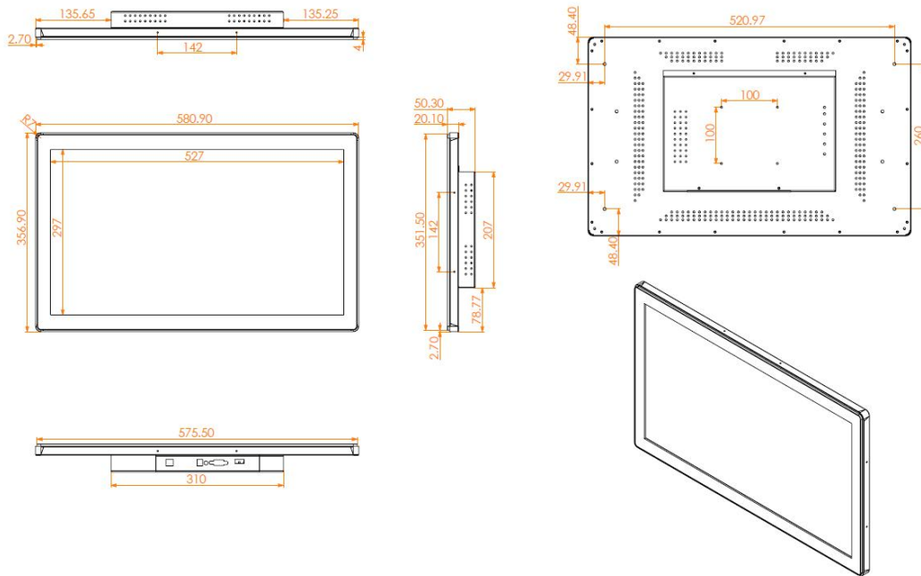
23.8寸尺寸示意图
