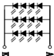
LED线路图(4串3并)
