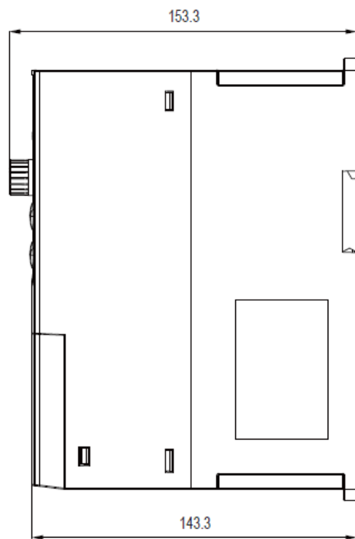
3.7kW—5.5kW 结构示意图及尺寸
