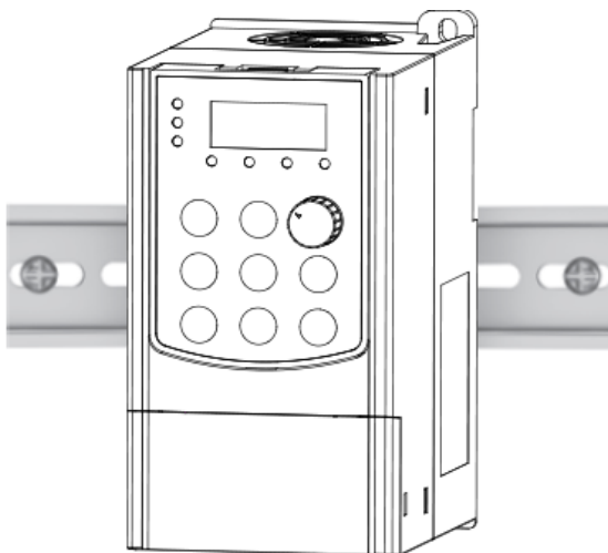
(2) 导轨式安装(仅限 7.5K 以下机种)
