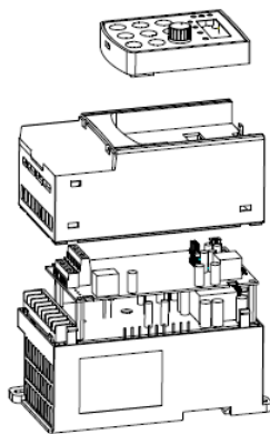
STEP 2 先拆卸按键面板组件， 再拆卸上盖
