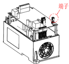
STEP 3 拔出风扇端子
