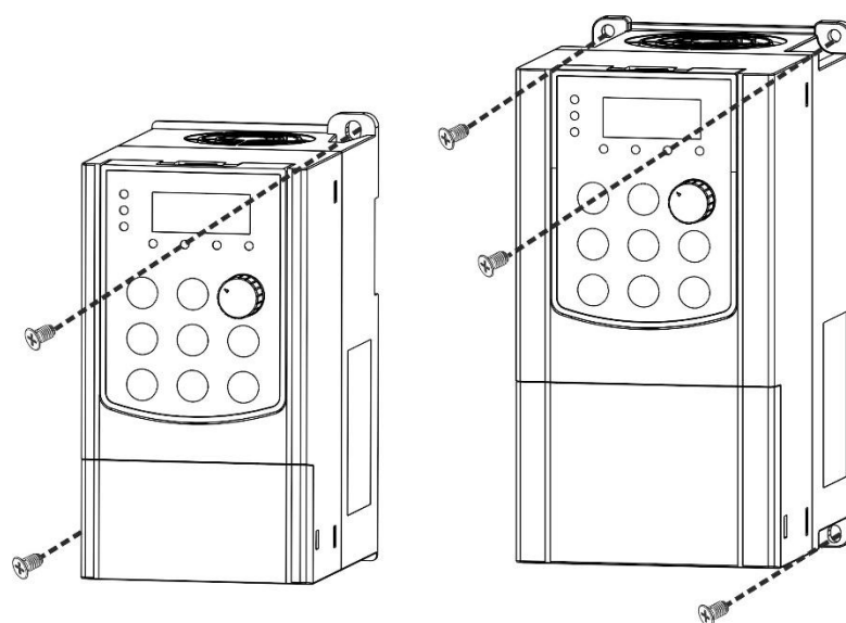
(1) 壁挂式安装
