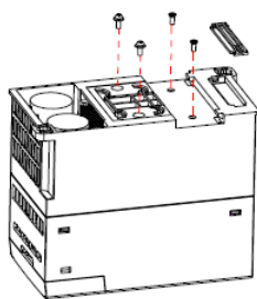
STEP 1 拆卸螺丝与风扇挡板
