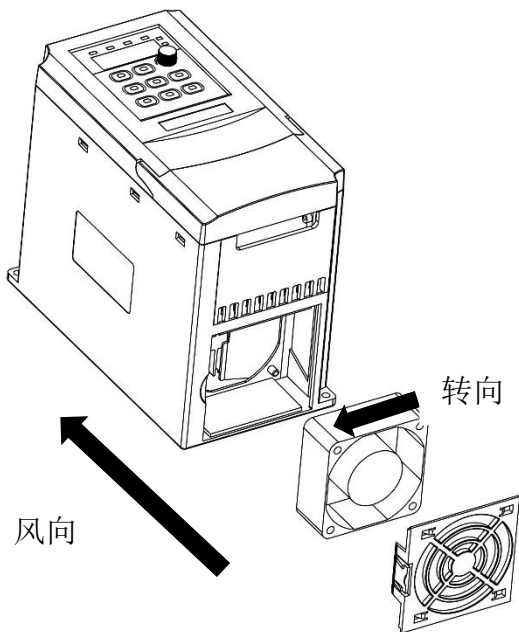
三相 380V 2.2KW 机器风扇维护示意图
