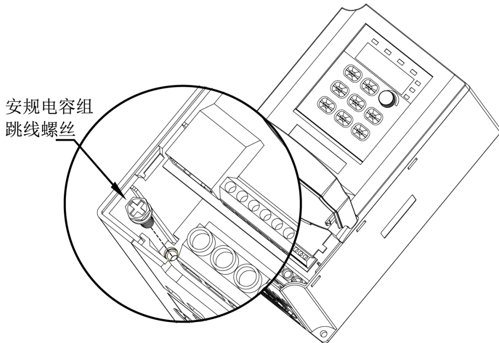
安规电容(EMC)对地跳线位置示意图
