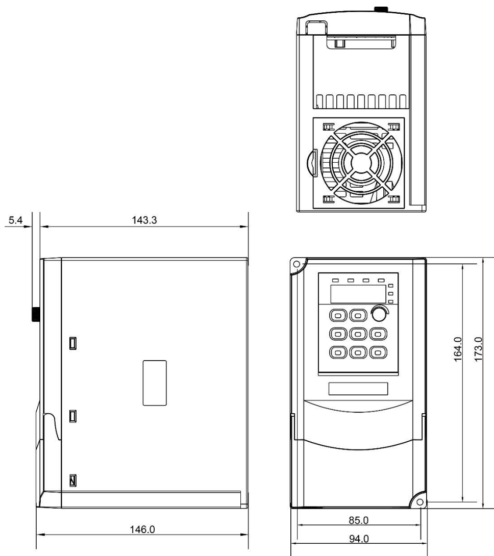
0.75KW—3.7KW 结构示意图及尺寸
