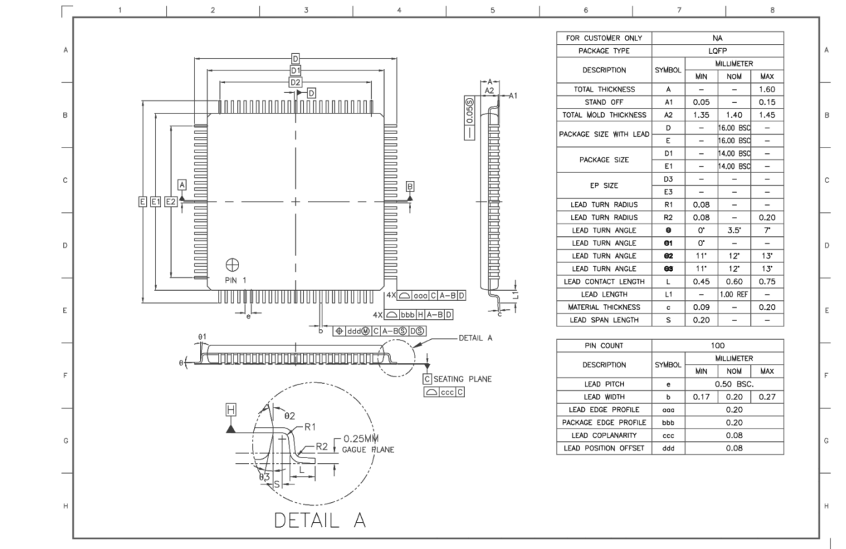
LQFP-100
