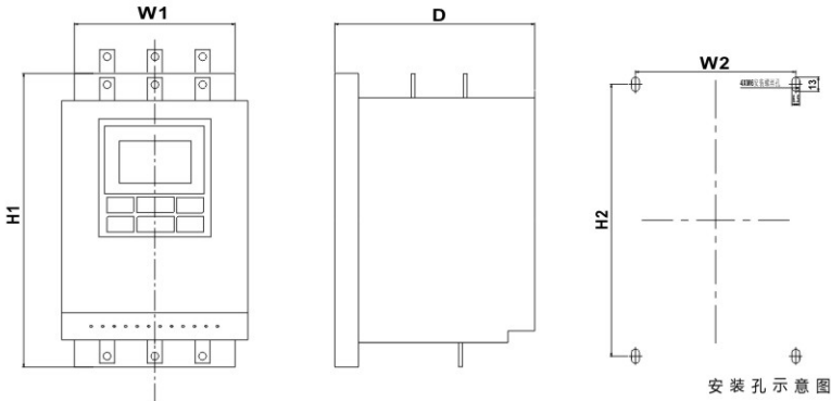
5.5kW ~ 600kW外型尺寸图
