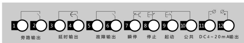
图4.3-1 外控端子图
