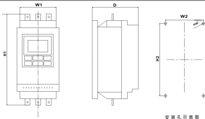
5.5kW ~ 600kW外型尺寸图
