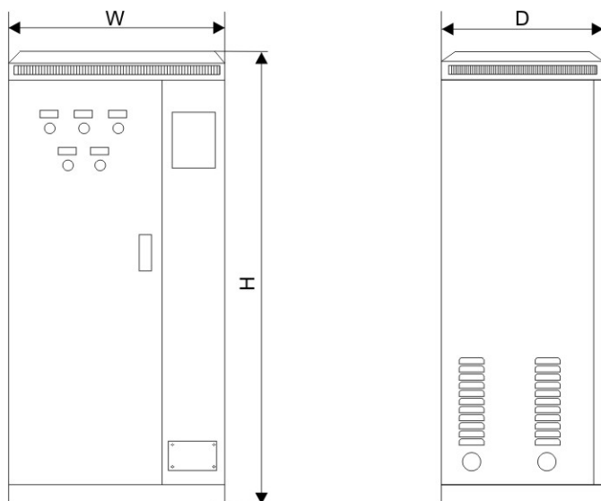
22kW~630kW外型尺寸图
