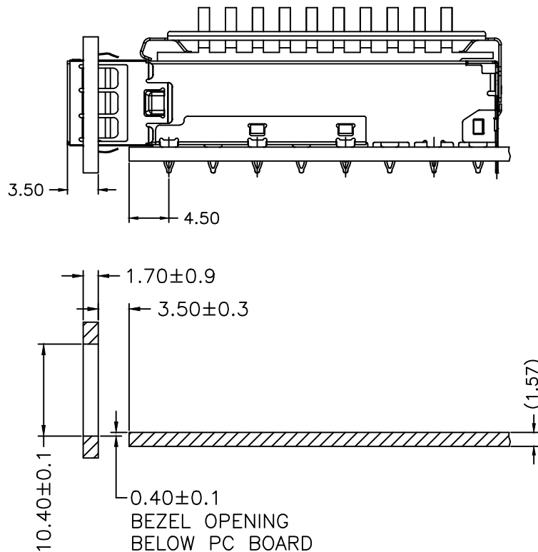
SECTION A-A
