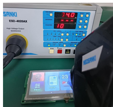
3.1 静电放电测试图
