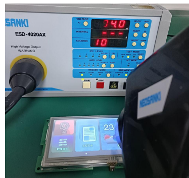
3.1 静电放电测试图
