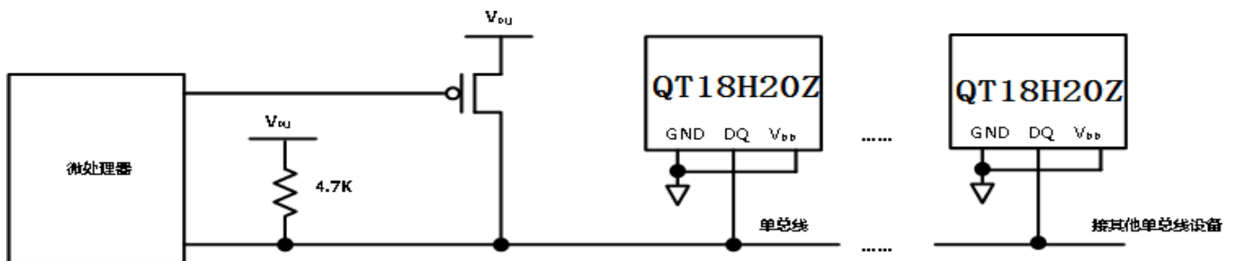
图 2: QT18H20Z 组网及寄生电源供电模式示意图
