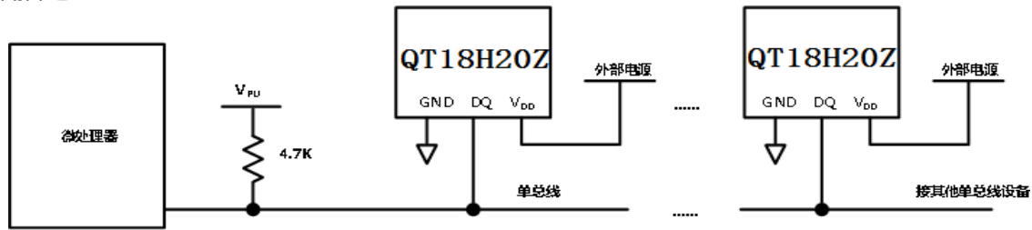
图 1: QT18H20Z 组网及外部电源供电模式示意图
