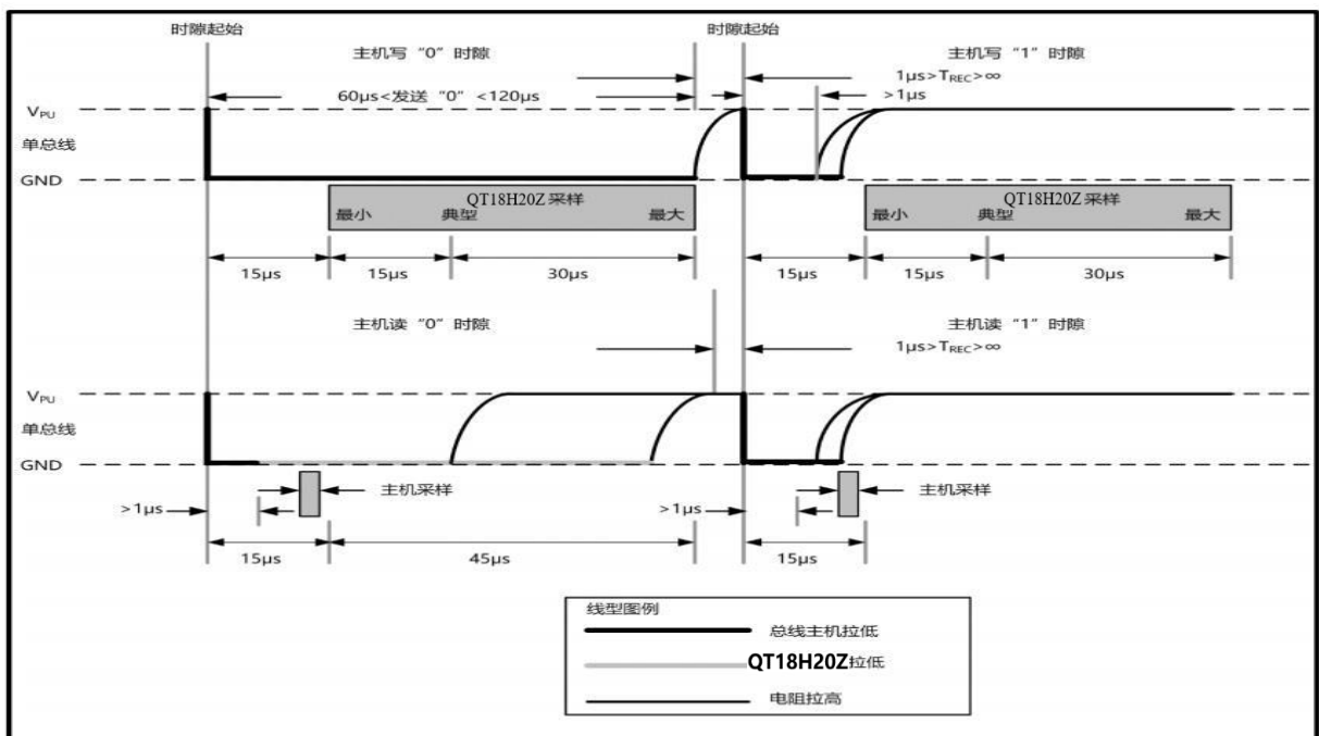
读/写时隙时序
