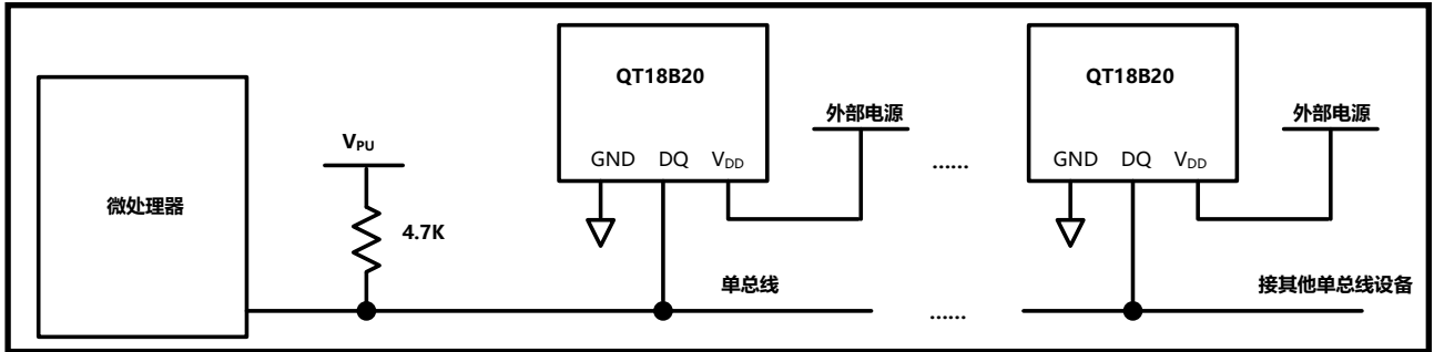
图 1: QT18B20 组网及外部电源供电模式示意图
