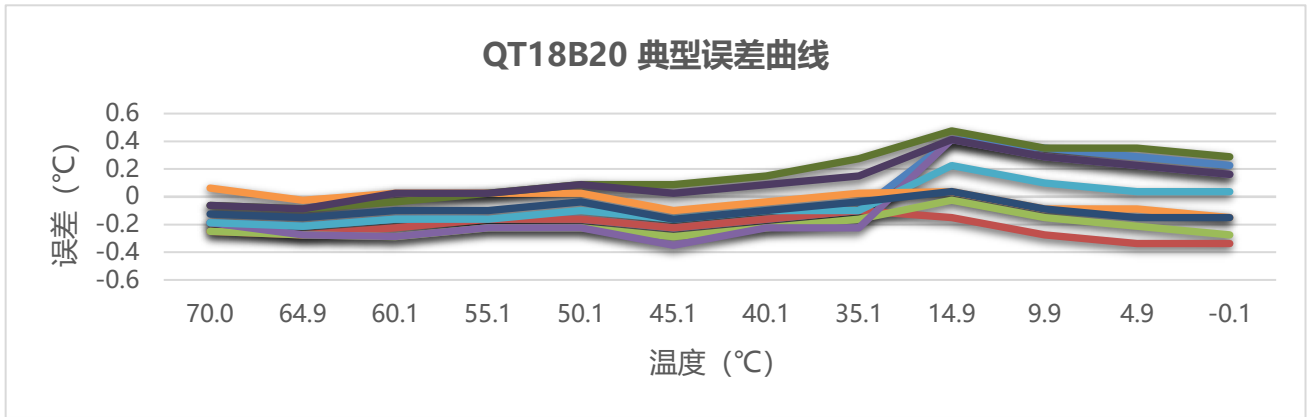
图 3: 典型误差曲线图
