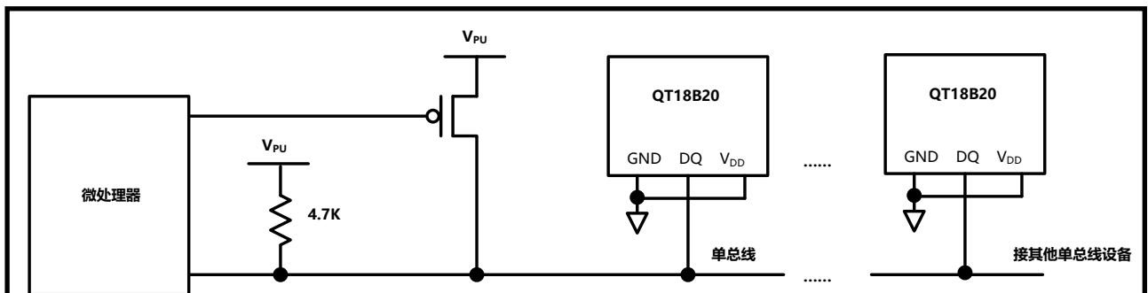
图 2: QT18B20 组网及寄生电源供电模式示意图
