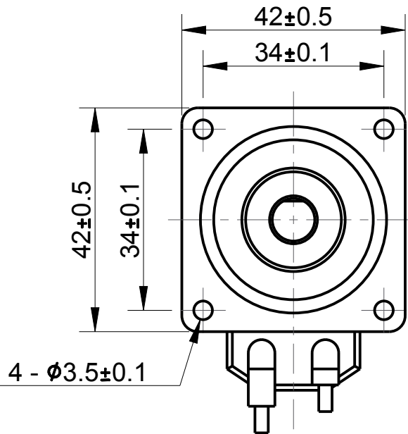
电机外形尺寸图 (DIMENSIONS)
