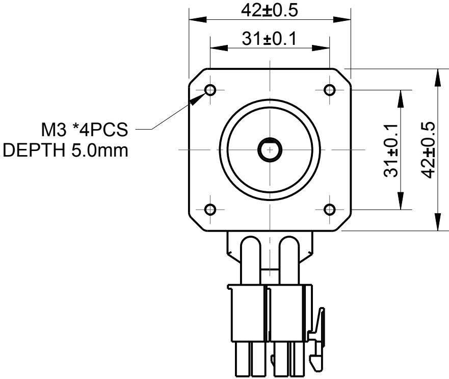
电机外形尺寸图 (DIMENSIONS)
