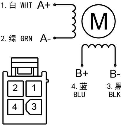
电气接线图 (Wiring Diagram)
