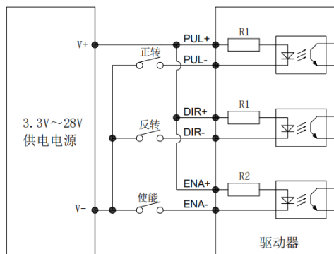
开关或继电器的连接方式，仅适用于I/O控制模式
