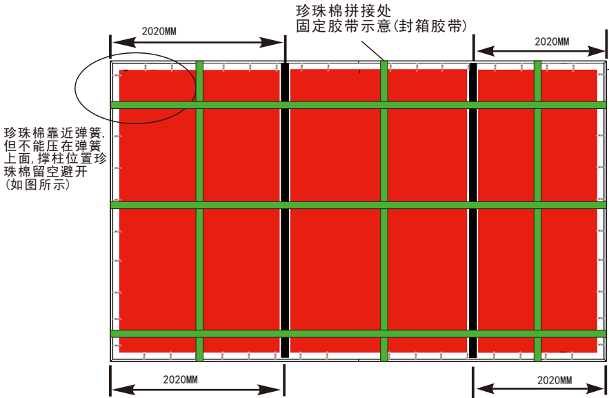
150寸以下珍珠棉安装图(棉为两层, 偏小的5MM层贴近感应层)
