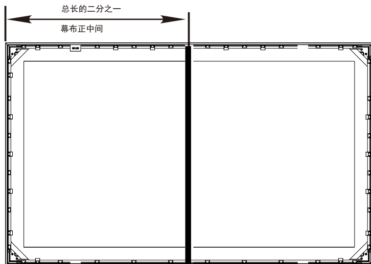
150寸以下撑杆安装图
