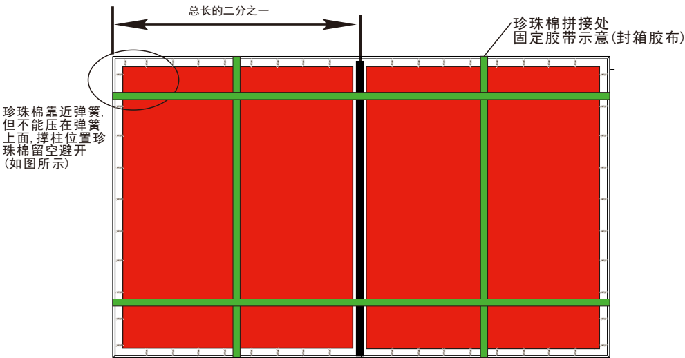
150寸以下珍珠棉安装图(棉为两层, 偏小的5MM层贴近感应层)
