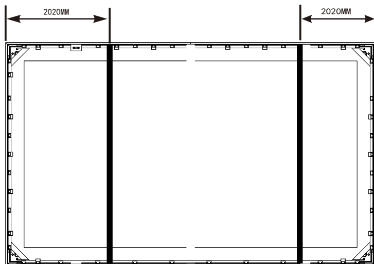
248寸撑杆安装图
