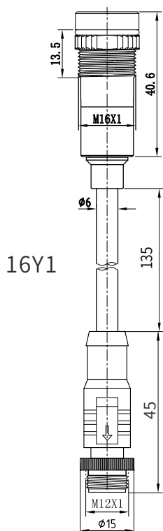
大手柄 方便操作 Big Handle
