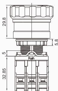
M3急停(铝氧化红色头部)
