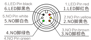
6线单色脚位
