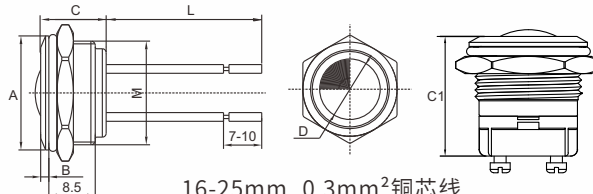
16-25mm 0.3mm 2 铜芯线 Copper core wire
