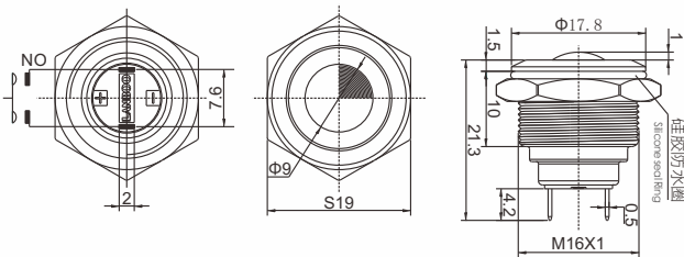
16E外形尺寸 Outline Dimension
