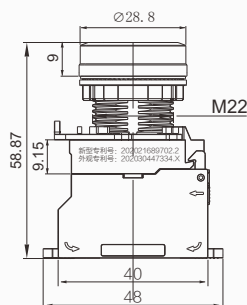
带灯自锁/自复 无灯自锁款
