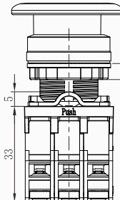
M4蘑菇头按钮(红色/绿色塑料头部)
