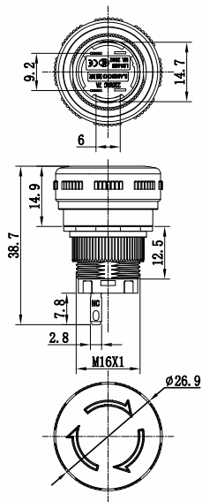
防滑头部设计 Head anti slip design
