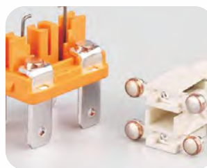
4颗加粗银触点 Silver Contact
