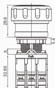
M1急停(塑料红色头部)
