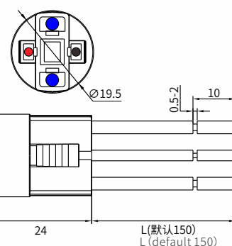
专用接插件 Connector
