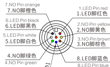
8线三色脚位
