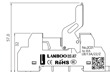
带测试扳手 Test wrench
