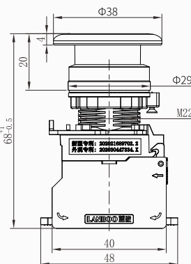
M4蘑菇头按钮(红色/绿色塑料头部)
