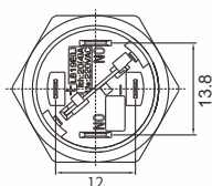
无极LED灯珠, 大触点 Non-Polar LED
