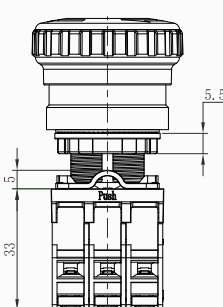
M2急停(塑料红色头部)
