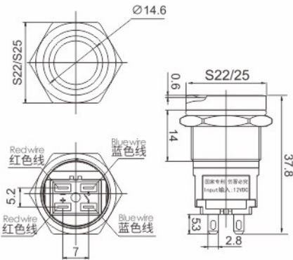
专用插件,卡扣设计 Connector
