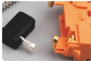
加粗触点,通过电流更大 Big Contact
