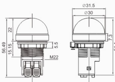
球头指示灯
