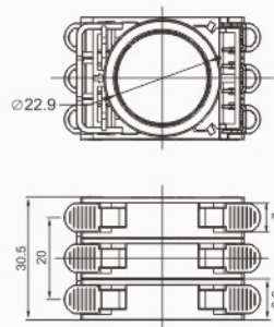
所有触点模块尺寸相同
