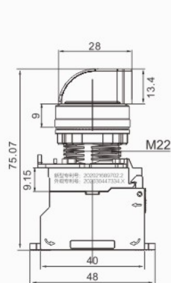
旋钮
