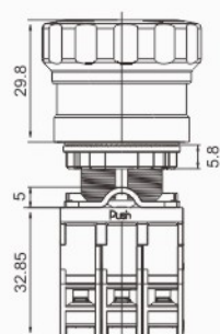
M3急停(铝氧化红色头部)
