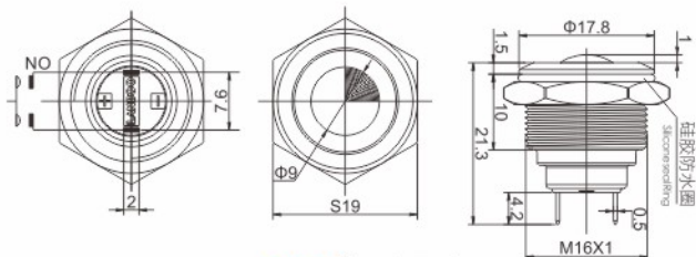
16E外形尺寸 Outline Dimension
