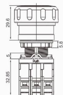
M1急停(塑料红色头部)
