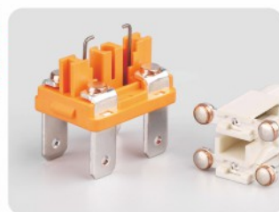
加大银点, 双锁钩 Bold Silver Contact
