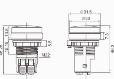
平头指示灯
