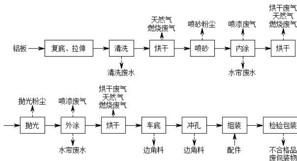
图 2-5 本项目生产工艺流程图
